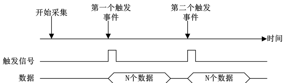
图 5-4-7 后触发和延时触发的重复触发
