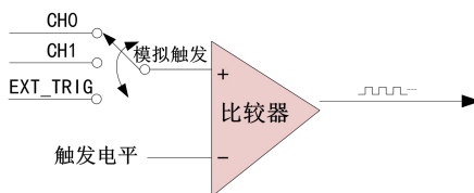
图5-3-4 比较器
