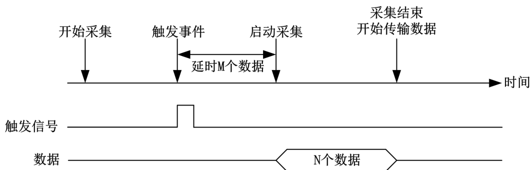
图 5-4-6 硬件延时触发
