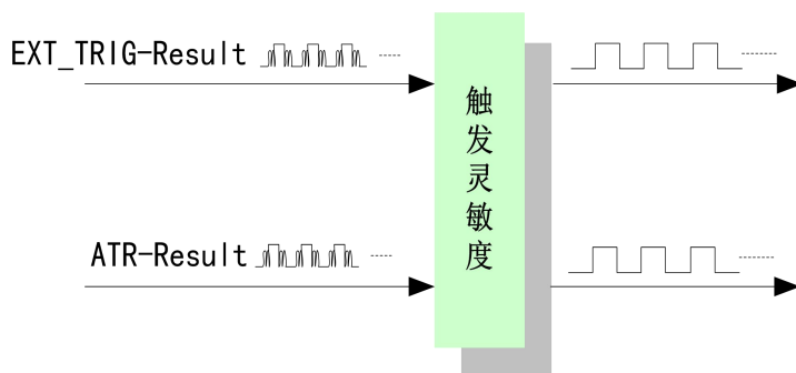
图 5-1-2 触发灵敏度
