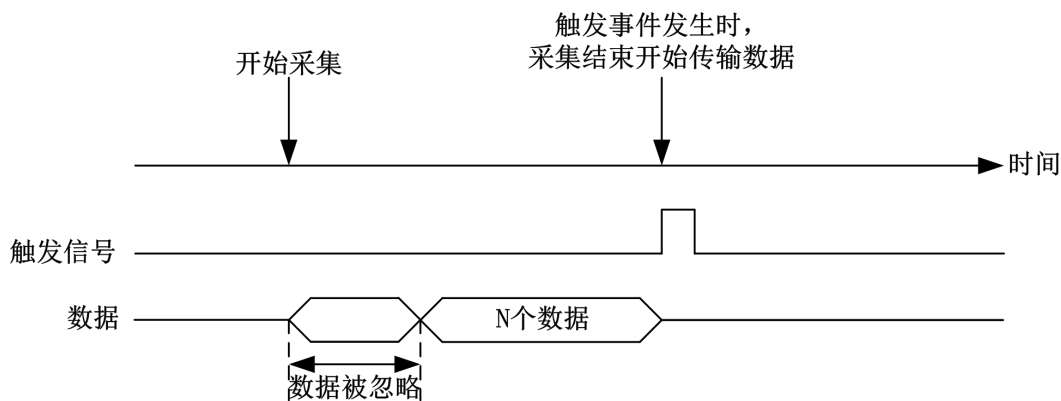
图 5-4-4 预触发
