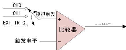
图5-3-2 模拟触发比较器
