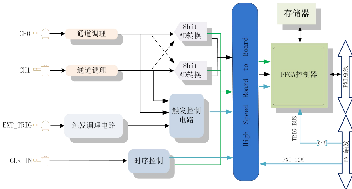
图 3-1-1 PXI8910 系统框图
